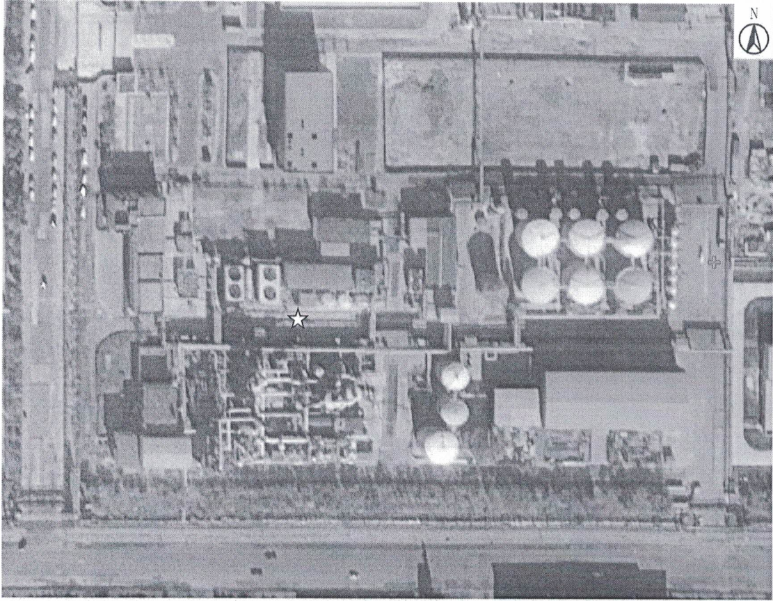
☆为废水采样点位
